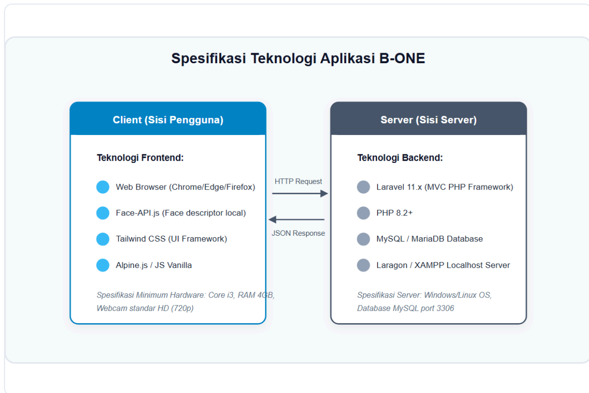
Gambar 2. Spesifikasi Teknologi Aplikasi B-ONE
